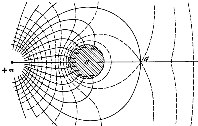
Abb. 24. Kraftlinien und Niveaufächen zweier ungleichnamigen Ladungen von verschiedener Größe.
